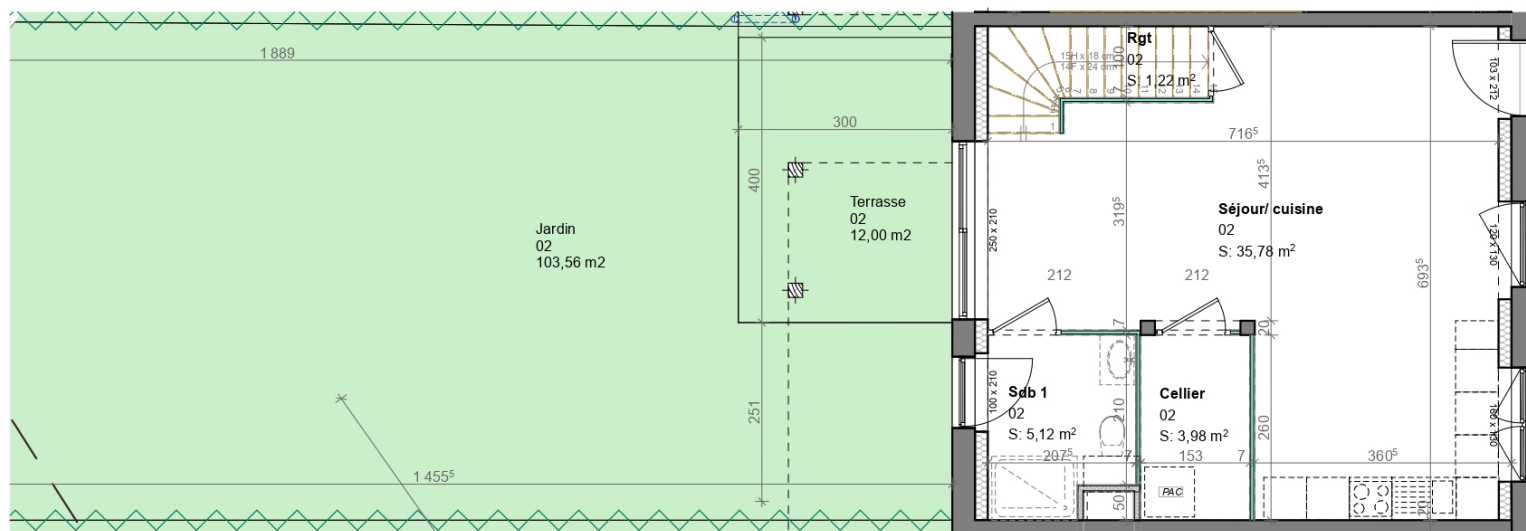
Rez-de-chaussée
