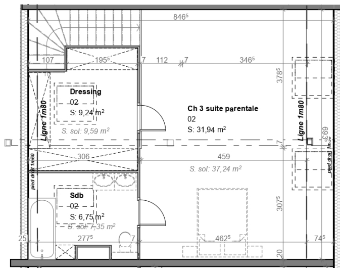
Comble
