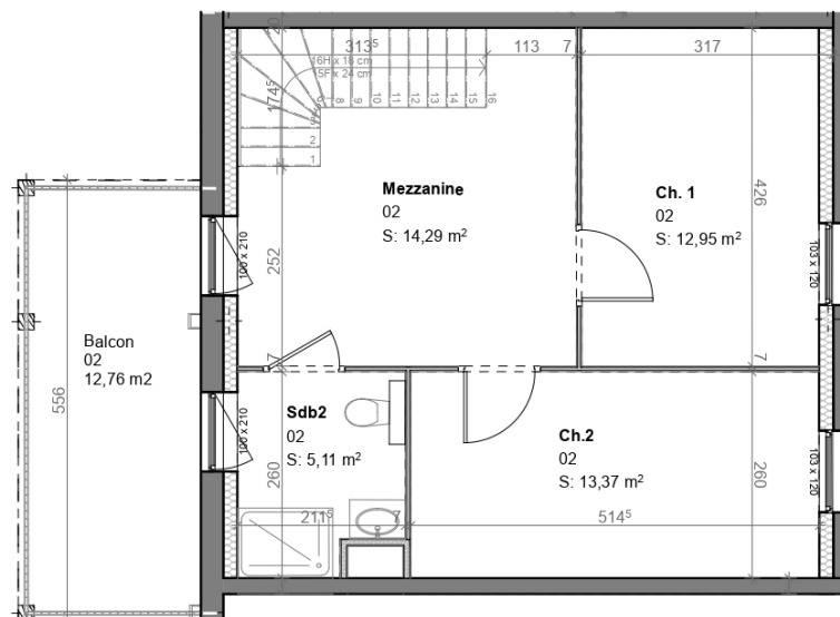
1er étage
